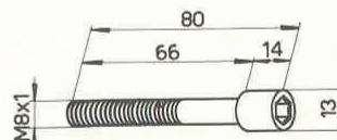
Vis 120VM-1203
