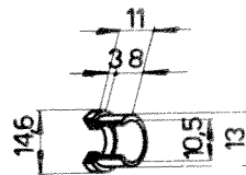
Douille 51-7013
