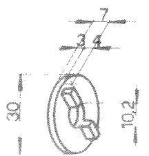
Arrêt 120-TS-100
