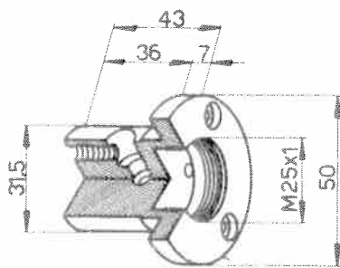
Corps de pompe 102VM-6157
