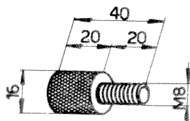
Vis de réglage 102-VM-24
