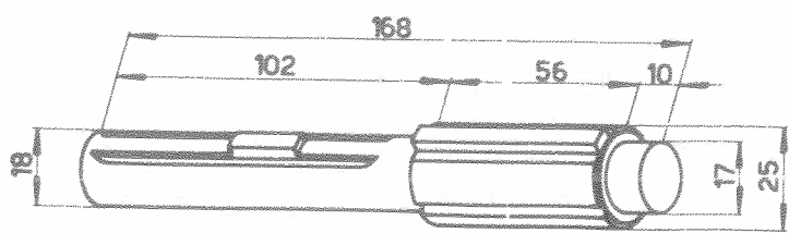
Arbre 102VM-6150
