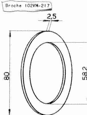
Fil. dents de scie. Pas 6 filets sur 10mm = 1,666
