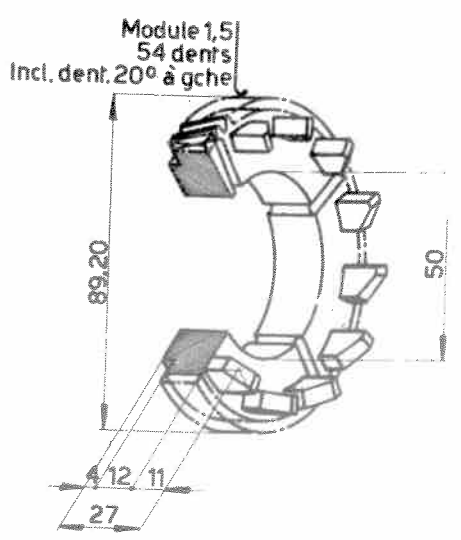
Roue hélicoïdale 102VM-6035
