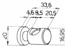
Tirant 102-605-S1
