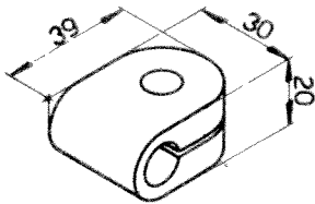
Bride 150-1401
