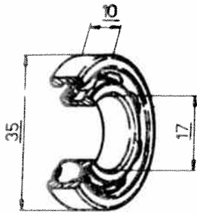
Roulement à billes SKF 6003X
