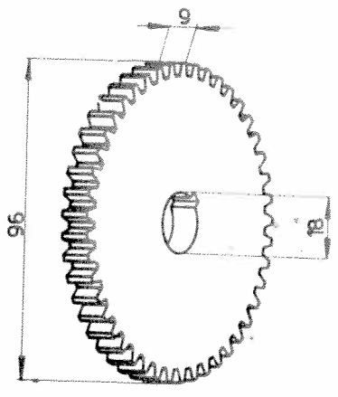
Roue dentée 102VM-6041
