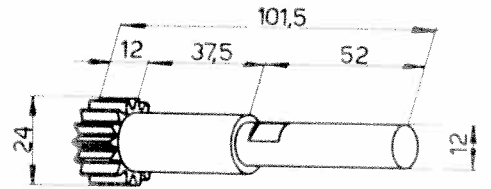
Pignon 102VM-760
