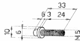
Vis pour lardon 11-33
