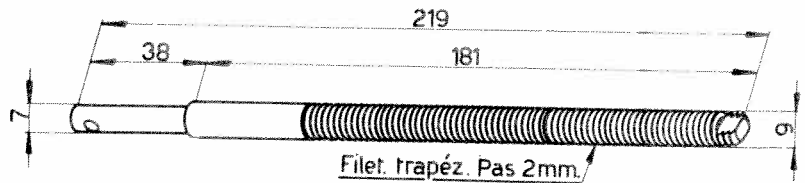
Vis supérieure 102VM-191
