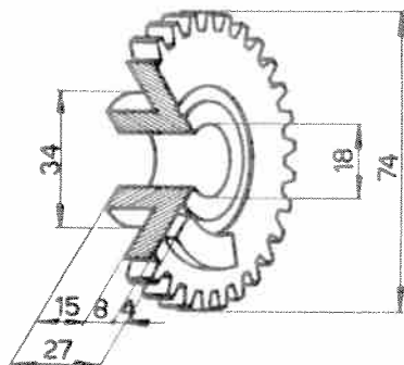
Roue dentée 102VM-6063
