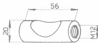
Fige de serrage 102VM-6066
