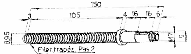
Vis 102-C-3
