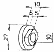
Rondelle à portée 102VM-1711
