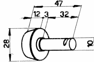
Axe 102VM-6083
