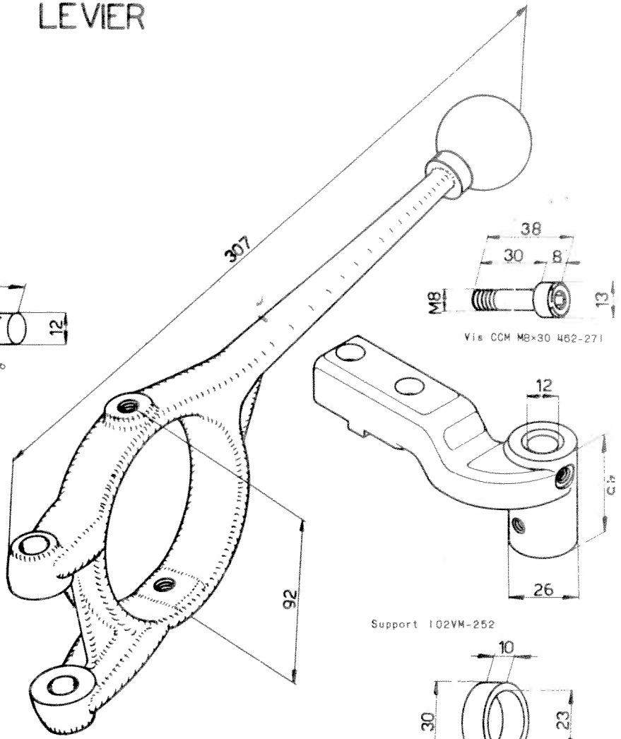
Levier 102-616-Q avec boule 463-410 C36n
