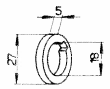
Bague intermédiaire 102VM-1714
