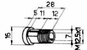
Douille 102-606-N
