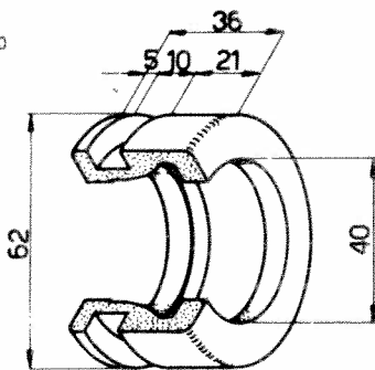
Bobine 102-616-V2
