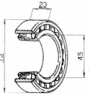
Roulement à rouleaux SKF NN3009K-C021
