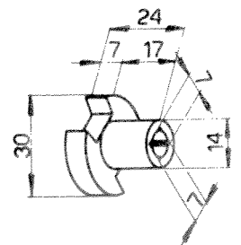
Entraîneur 102-G-2
