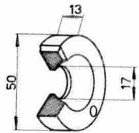
Bague à rotule 102VM-683
