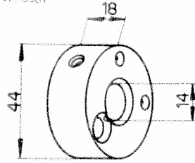
Disque 102VM-6073
