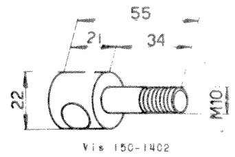
Vis 150-1402
