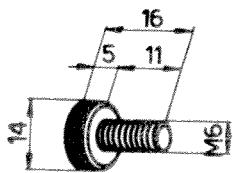
Vis E M6x11 462-275
