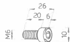
Vis CCM M6x20 462-270
