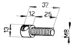
Vis de blocage 102-VM-791
