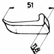
Chien 120-P-109
