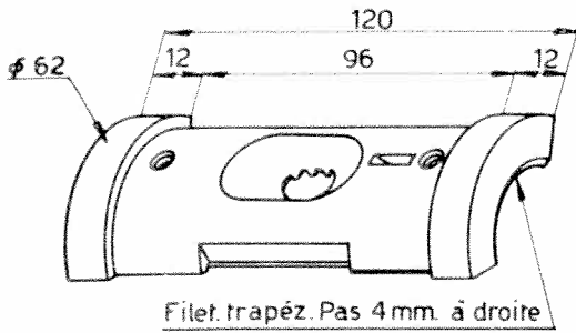
Peigne 102VM-704
