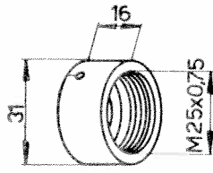
Ecrou-repère 102-608-Y
