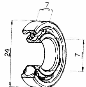
Roulement à billes 102-CH-170
