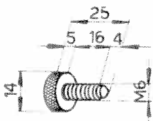
Vis 102VM-737
