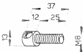
Vis de blocage 102VM-791
