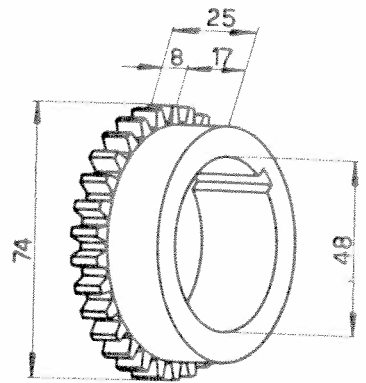
Roue dentée 102VM-6096
