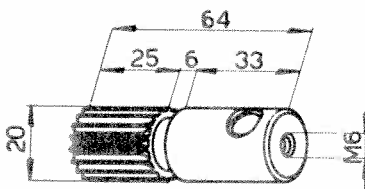
Pignon 102VM-788
