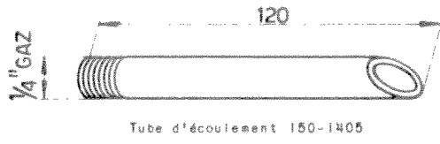
Tube d'écoulement 150-1405
