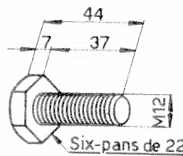
Vis 102VM-6094
