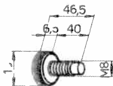
Vis E2 M8x40 462-277
