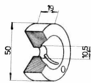
Bague à rotule 102VM-685
