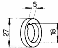
Bague Intermédiaire 102VM-1714
