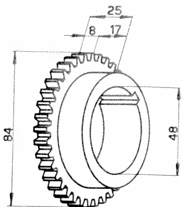
Roue dentée 102VM-6036
