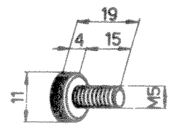
Vis E M5x15 462-274
