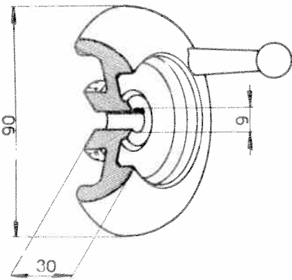
Volant 102VM-353 Poignée 463-402 8x14x55
