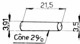
Goupille conique 102-CH-192 Ech: 2:1
