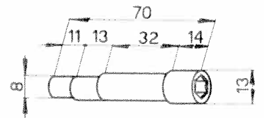
Excentrique 102VM-356
