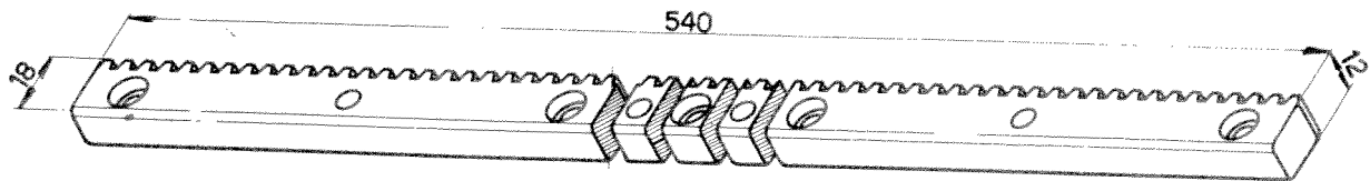
Crémaillère 102-VM-8
