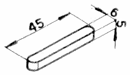
Clavette 102VM-6098
