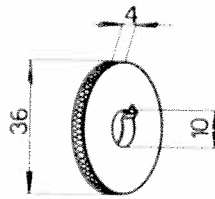
Rondelle 102VM-1303
