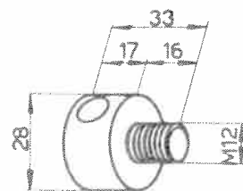
Vis de blocage 102VM-6047
