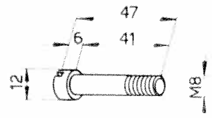
Vis-garde 102VM-705
