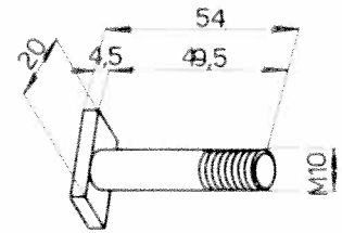
Tige de blocage 102-VM-1392
