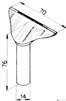
Eventail 102-615-B
