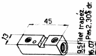
Ecrou supérieur 102-CH-133
