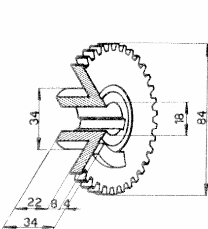
Roue dentée 102VM-6062
