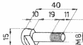
Vis de fixation 102-618-C
