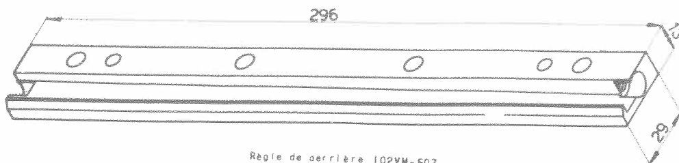
Règle de derrière 102VM-807
