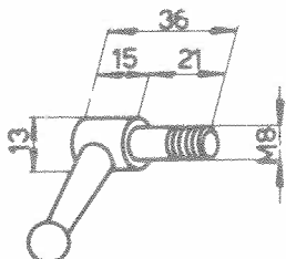
Vis de blocage 102VM-141 Poignée M63-402 8x10x45
