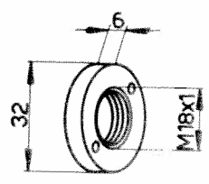
Ecrou 102VM-6042
