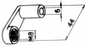
Levier division 102-605-B
