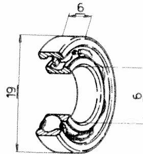
Roulement à billes SKF EL6
