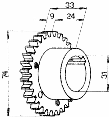
Roue dentée 102VM-104
