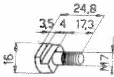
Vis de fixation 102-611-L
