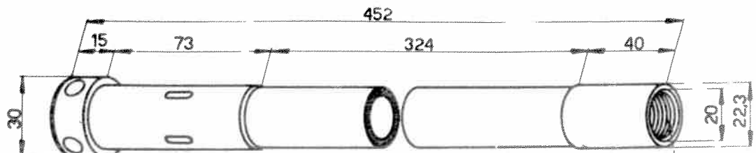
Fil.dents de scie. Pas 6 filets sur 10mm=1,666
