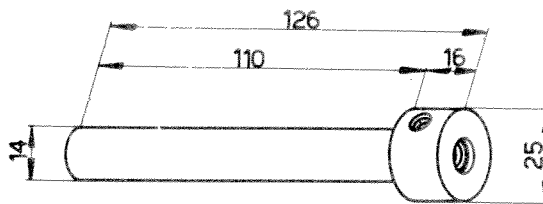
Bouée 102-VM-22
