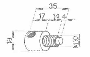
Arbre 102VM-6113
