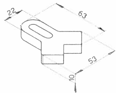
Chien 102VM-1652
