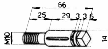
Tourillon 102VM-1712
