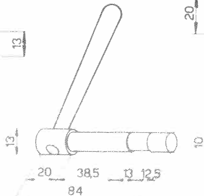
Excentrique 102-608-J Manette 463-400 7x10x60
