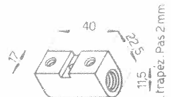
Ecrin inférieur 102VM-727
