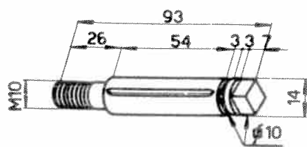
Tourillon 102VM-1720
