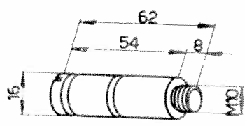
Guide 102VM-6044
