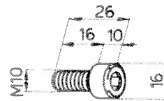
Vis OCM M10x16 162-270
