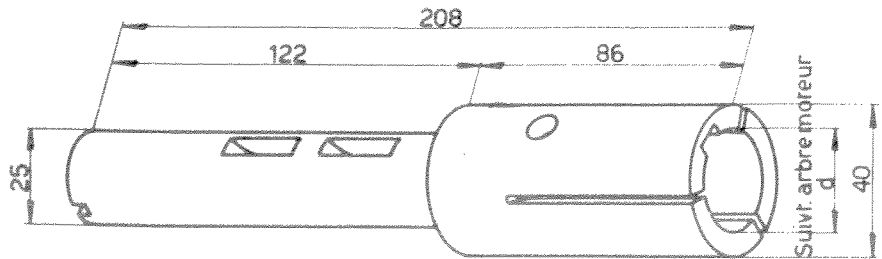
Arbre 120-TS-38
