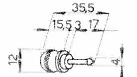
Tige pour huile 102-608-V
