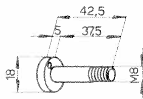
Tige de fixation 102VM-1655
