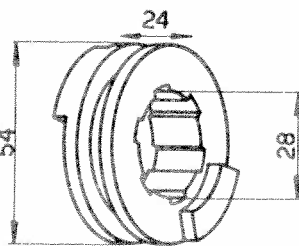
Entraineur 102VM-6152
