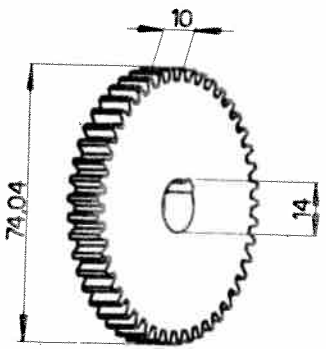
Roue dentée 102VM-6081
