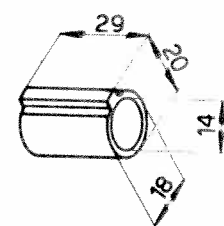
Douille à ergot 102VM-1713
