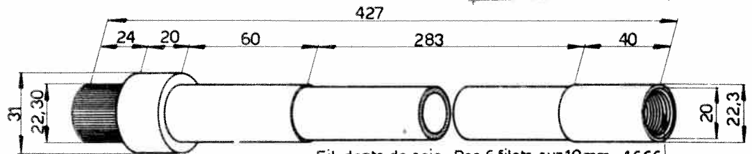
Fil. dents de scie. Pas 6 filets sur 10mm = 1,666
