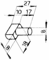
Doigt 102VM-6070
