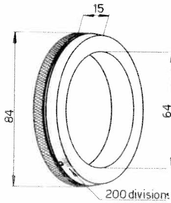
Vernier 102VM-733
