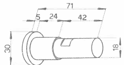
Tourillon 102VM-6064
