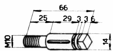
Tourillon 102VM-1712
