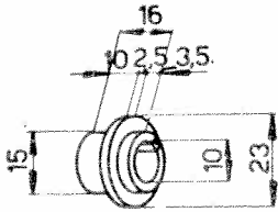
Douille 102-608-P
