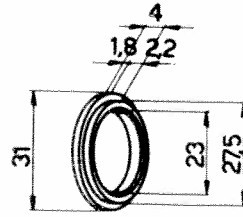
Bague 102-P20-10
