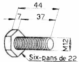
Vis 102VM-6094
