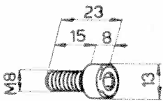
Vis OCM M8x15 162-270
