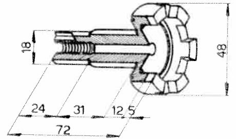
Arbre porte-engrenage 102VM-6147
