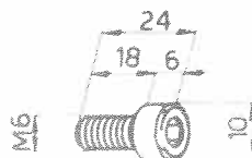
Vis OCM M6x16 162-270
