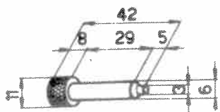
Piston 102-605-P
