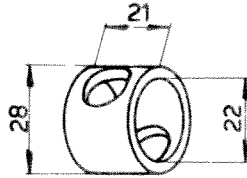
Douille 51-7025
