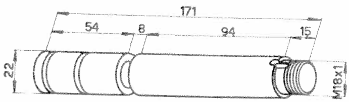
Arbre 102VM-6040
