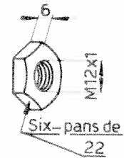
Contre-écrou spécial 102VM-736
