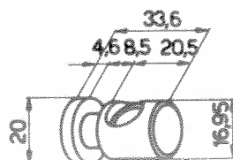
Tirant 102-605-S1
