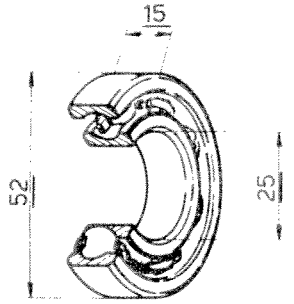
Roulement à billes SKF 6205
