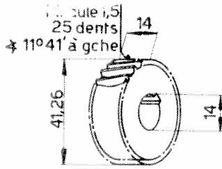
Roue hélicoïdale 102VM-6067
