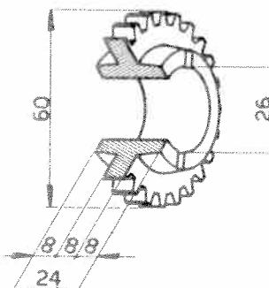
Roue intermédiaire 102VM-6065
