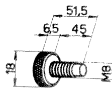
Vis E2 M8x45 462-277
