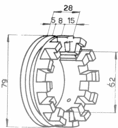
Entraîneur 102VM-6032
