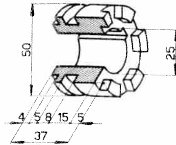
Entraineur 102VM-6057
