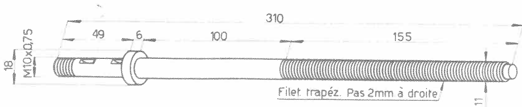
Vis 102VM-725
