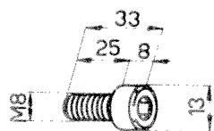
Vis CCM M8x25 462-270
