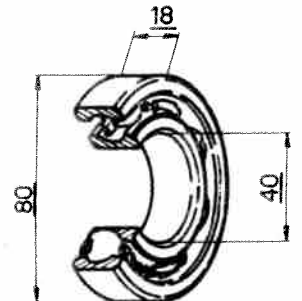
Roulement à billes SKF 6208-C153
