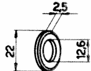
Rondelle 102-606-R
