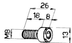
Vis CCM M8x18 462-270
