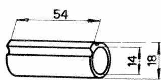
Douille à ergot 102VM-1721
