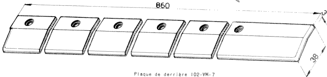
Plaque de derrière 102-VM-7
