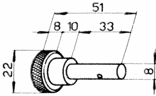
Poullet 120VM-11
