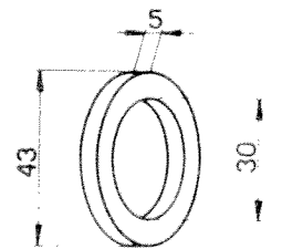
Rondelle feutre SKF Fi 7
