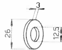
Rondelle 102VM-6095
