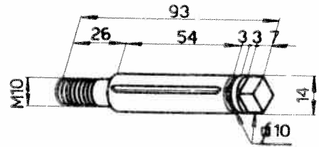
Tourillon 102VM-1720
