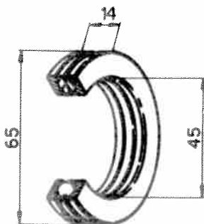
Butée à billes SKF 51109-C05
