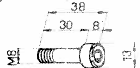
Vis CCM MBx30 462-271
