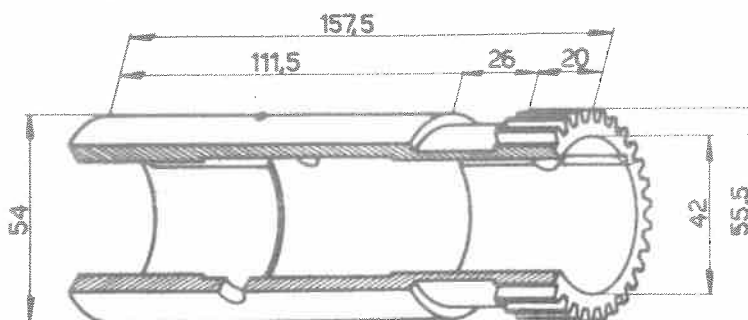
Douille 102VM-213
