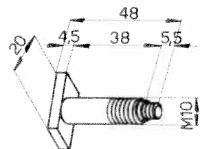
Tige de fixation 102VM-1602
