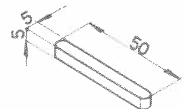
Clavette 102VM-6093
