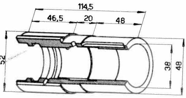
Douille 102VM-6033
