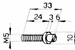
Vis 11A-504
