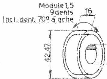
Roue hélicoïdale 102VM-6082
