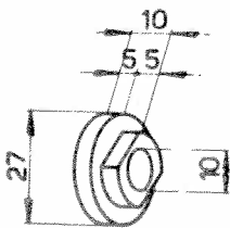
Rondelle à portée 102VM-1711
