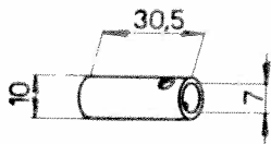
Douille 102-CH-187
