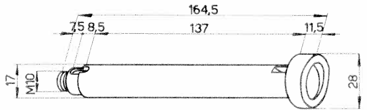
Axe 102VM-6155
