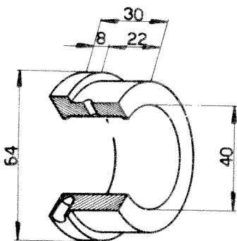
Douille 102-VM-226
