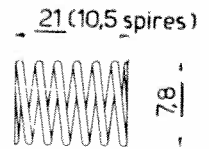
Ressort 0078-39
