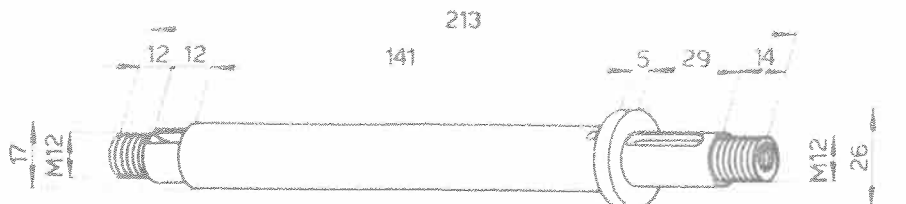
Arbre 102VM-6086
