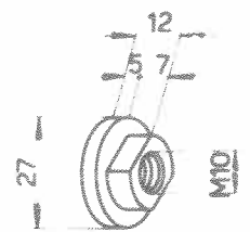
Ecrou 102VM-1710
